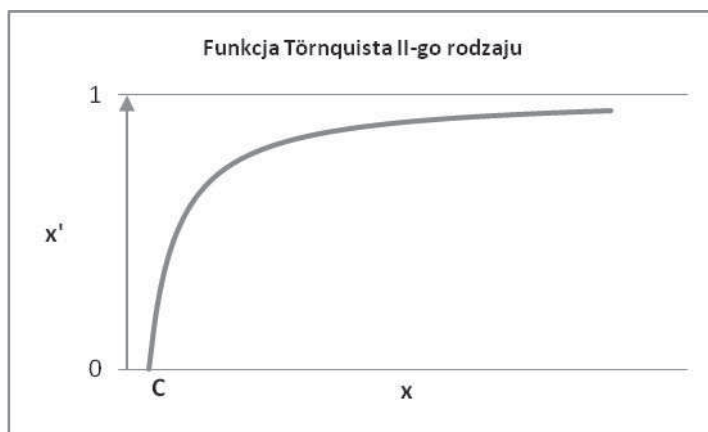
Rys. 4. Wykres funkcji Törnquista II rodzaju dla a=b=c=1
