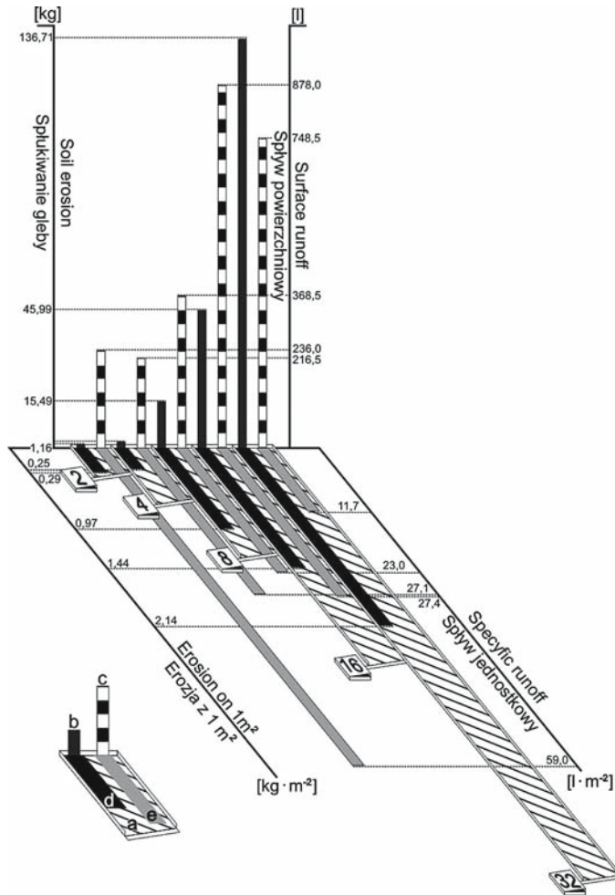
Ryc. 5. Spływ i splukiwanie gleby na poletkach o różnej długości użytkowanych jako czarny ugor [a – poletko doświadczalne, b – splukiwanie gleby (kg), c – spływ powierzchniowy ( \text{dm}^3 ), d – erozja z 1\text{m}^2 ( \text{kg}\cdot\text{m}^{-2} ), e – spływ jednostkowy ( \text{dm}^3\cdot\text{m}^{-2} )]
